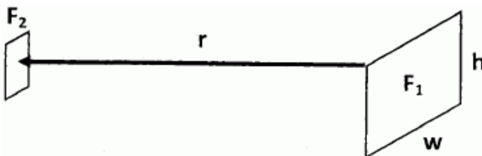
Рисунок А.3.1. Расположение излучающей поверхности пламени F_1 и облучаемой поверхности материала соседнего объекта F_2 ,
